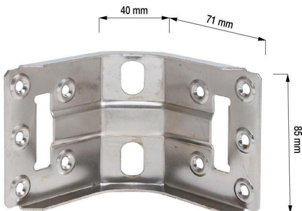
Angolare rinforzato - Misure: 85/40/71 Strengthened angle bracket - Measures: 85/40/71 Verstärkter Winkel - Maßen: 85/40/71
