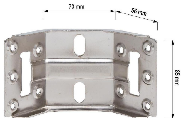
Angolare rinforzato - Misure: 85/70/56 Strengthened angle bracket - Measures: 85/70/56 Verstärkter Winkel - Maßen: 85/70/56
