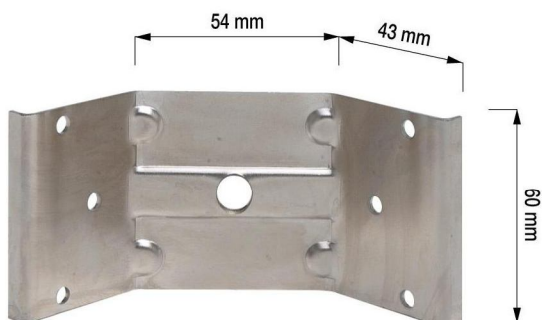
Angolare con foro centrale - Misure: 60/54/43 Angle bracket with central hole - Measures: 60/54/43 Winkel mit zentralem Loch - Maßen: 60/54/43 Cod. 2.01.003
