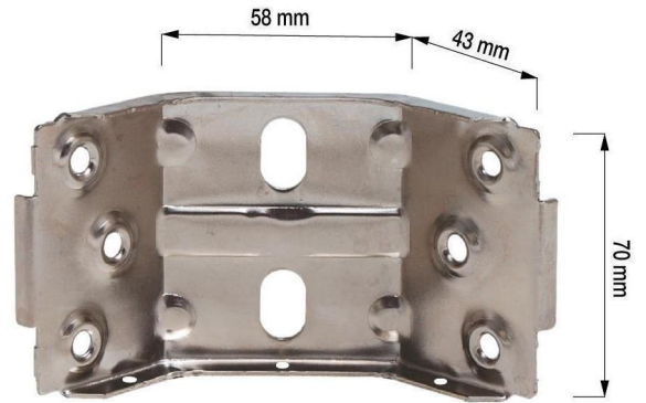
Angolare rinforzato con 3 fori Ø 3,2 mm - Misure: 70/58/43 Strengthened angle bracket with 3 holes Ø 3,2 mm Measures: 70/58/43 Verstärkter Winkel mit 3 Löcher Ø 3,2 mm Maßen: 70/58/43
