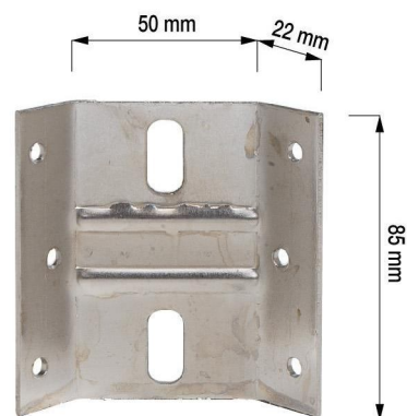
Angolare - Misure: 85/50/22 Angle bracket - Measures: 85/50/22 Winkel - Maßen: 85/50/22 Cod. 2.01.006.Z02
