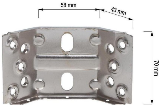
Angolare rinforzato con bugne con 3 fori Ø 3,2 mm Misure: 70/58/43 Strengthened angle bracket with juts with 3 holes Ø 3,2 mm Measures: 70/58/43 Verstärkter Winkel mit Ausbuchtungen mit 3 Löcher Ø 3,2 mm Maßen: 70/58/43
