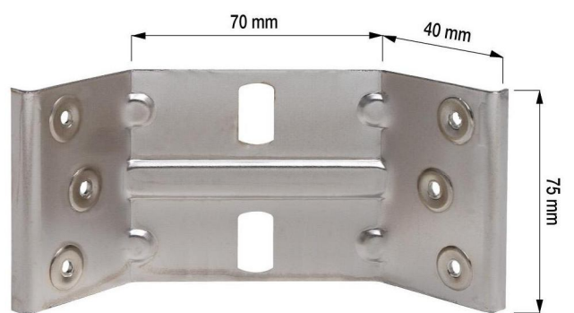
Angolare - Misure: 75/70/40 Angle bracket - Measures: 75/70/40 Winkel - Maßen: 75/70/40
