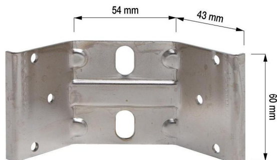
Angolare - Misure: 60/54/43 Angle bracket - Measures: 60/54/43 Winkel - Maßen: 60/54/43 Cod. 2.01.002
