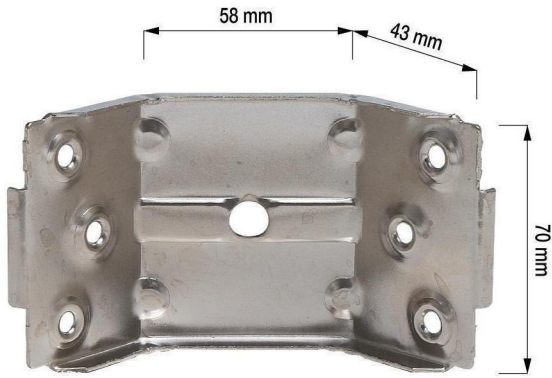
Angolare rinforzato con foro centrale - Misure: 70/58/43 Strengthened angle bracket with central hole - Measures: 70/58/43 Verstärkter Winkel mit zentralem Loch - Maßen: 70/58/43
