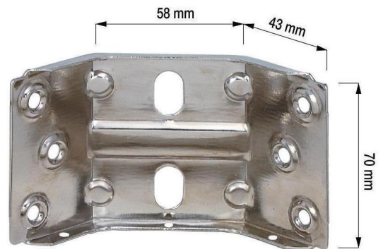
Angolare rinforzato senza bugne e senza pieghe con 3 fori Ø 3,2 mm - Misure: 70/58/43 Strengthened angle bracket without juts, fold, with 3 holes Ø 3,2 mm - Measures: 70/58/43 Verstärkter Winkel ohne Ausbuchtungen mit 3 Löcher Ø 3,2 mm - Maßen: 70/58/43
