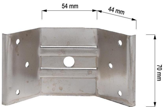
Angolare con foro centrale - Misure: 70/54/44 Angle bracket with central hole - Measures: 70/54/44 Winkel mit zentralem Loch - Maßen: 70/54/44
