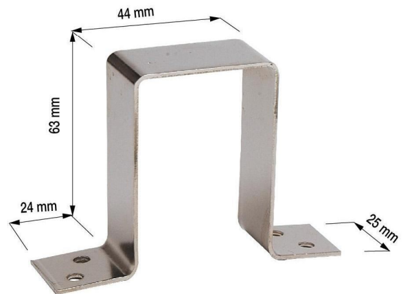
Cavallotto - Misure: 63/44/24 U-bolt - Measures: 63/44/24 Bügelbolzen - Maßen: 63/44/24 Cod. 2.03.005
