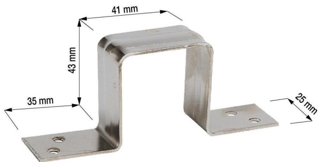
Cavallotto - Misure: 43/41/35 U-bolt - Measures: 43/41/35 Bügelbolzen - Maßen: 43/41/35 Cod. 2.03.004
