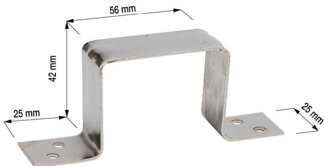
Cavallotto - Misure: 42/56/25 U-bolt - Measures: 42/56/25 Bügelbolzen - Maßen: 42/56/25 Cod. 2.03.003
