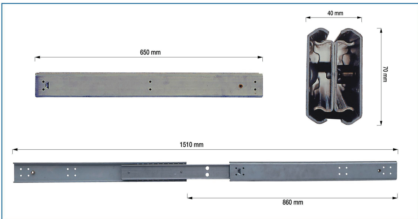
Guida telescopica. Telescopic slide. Teleskopische Führung.
