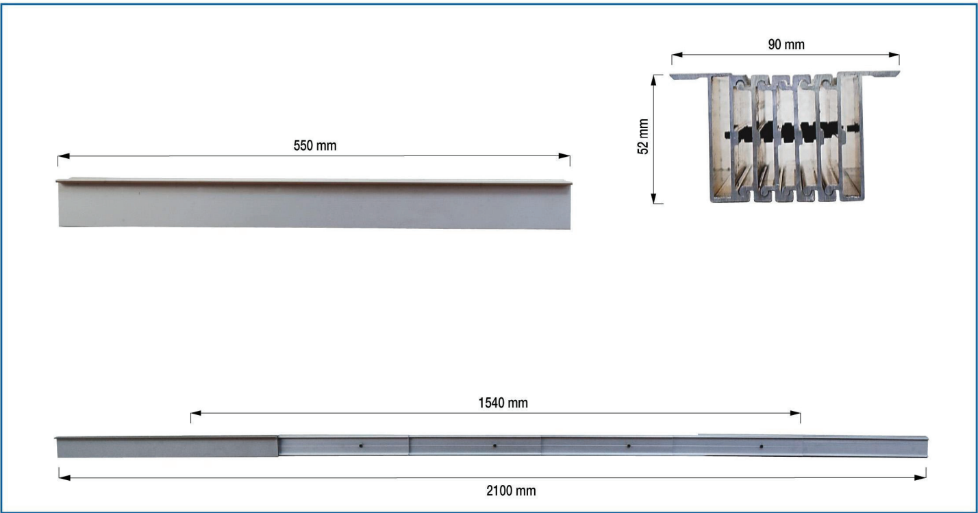
Guida telescopica alluminio. Aluminium telescopic slide. Teleskopische Führung aus Aluminium.
