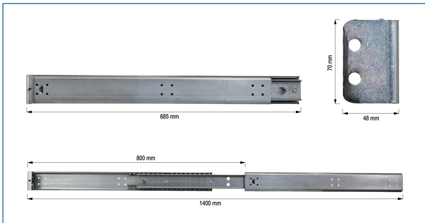
Guida telescopica con piastra saldata. Telescopic slide with welded plate. Teleskopische Führung mit geschweisster Platte.
