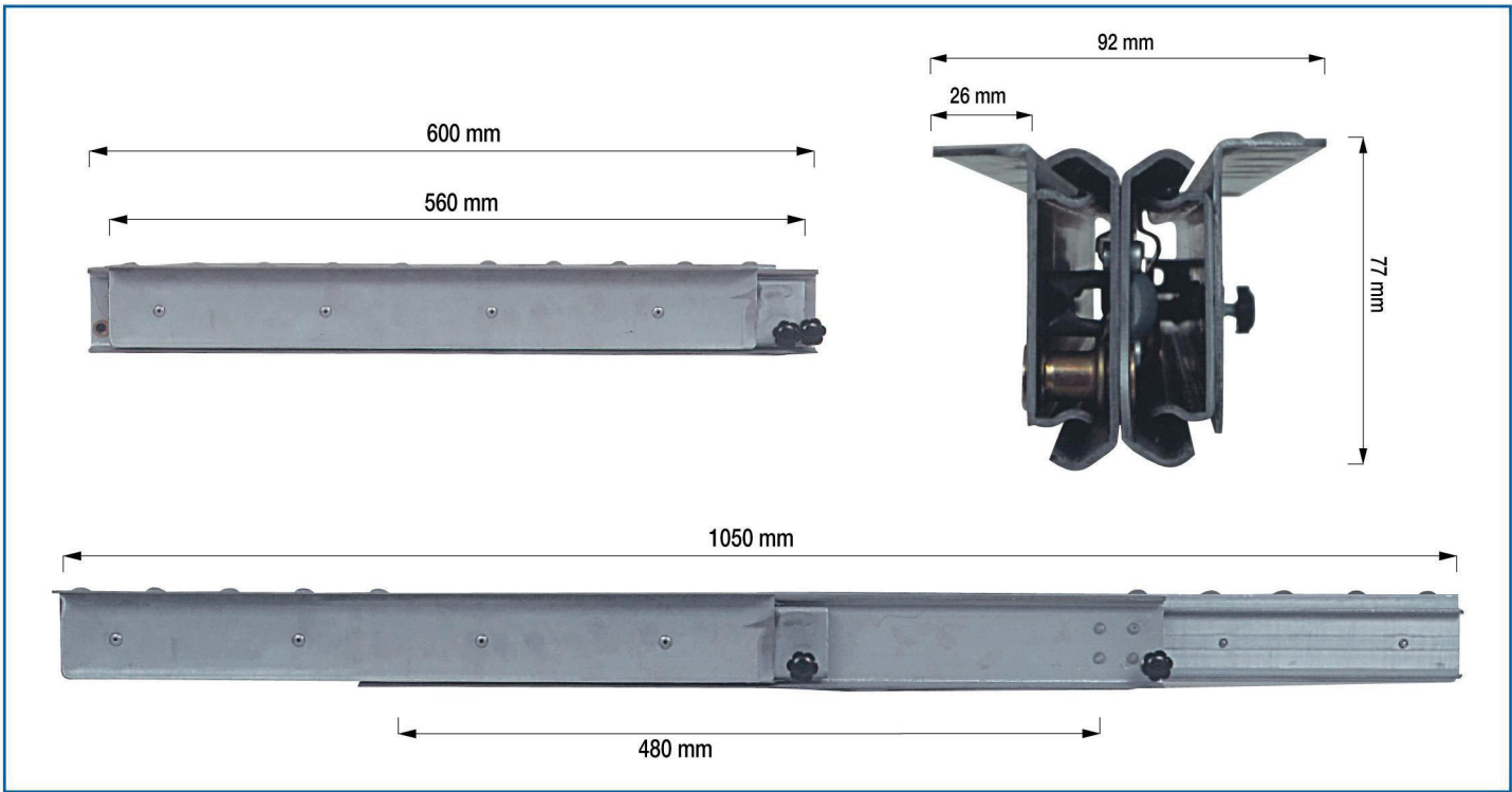
Guida telescopica con bloccaggio. Telescopic slide with locking system. Teleskopische Führung mit Arretierung.
