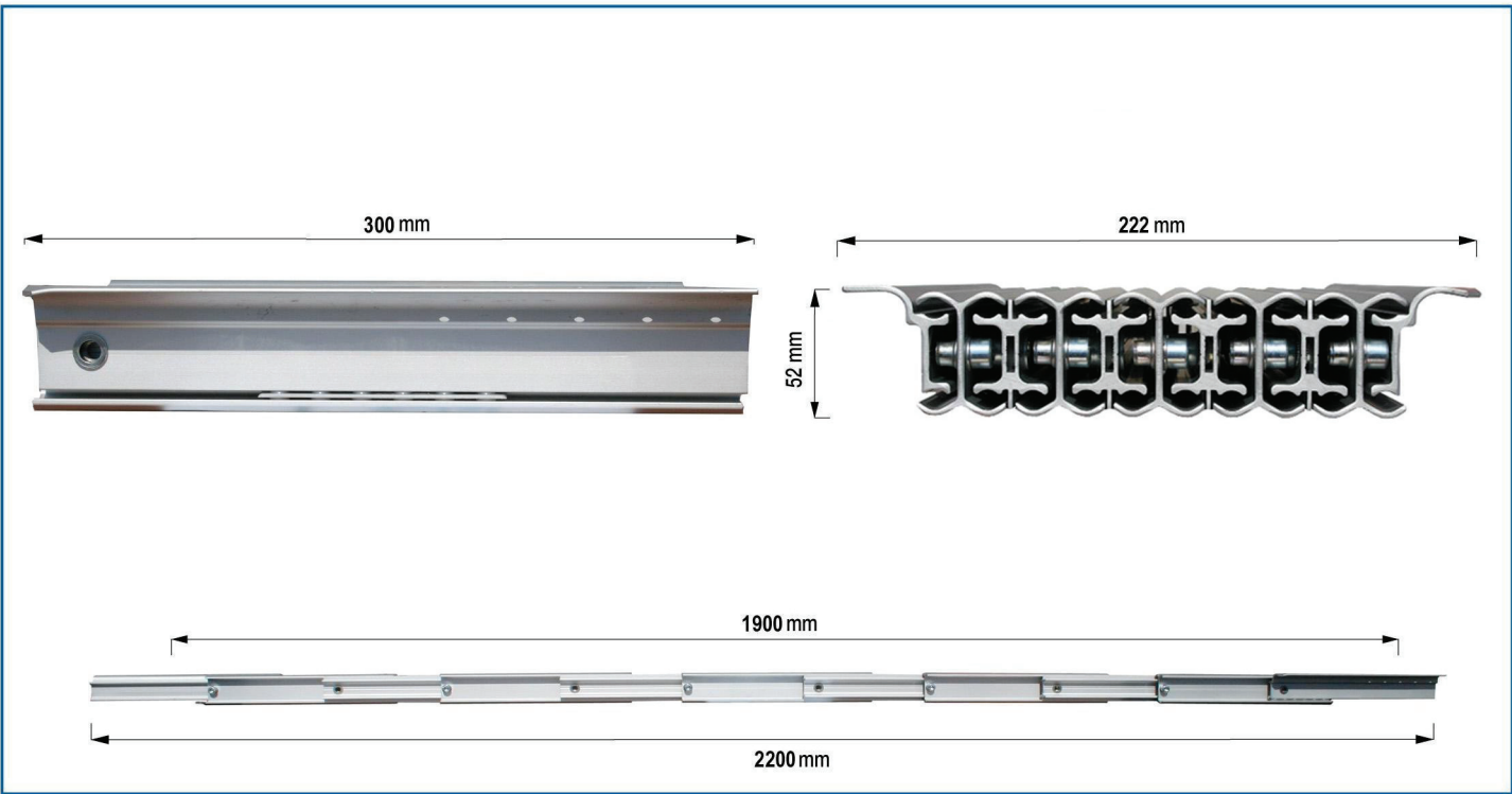
Guida telescopica in ferro o alluminio. Aluminium or iron telescopic slide. Teleskopische Führung aus Aluminium oder Eisen.
